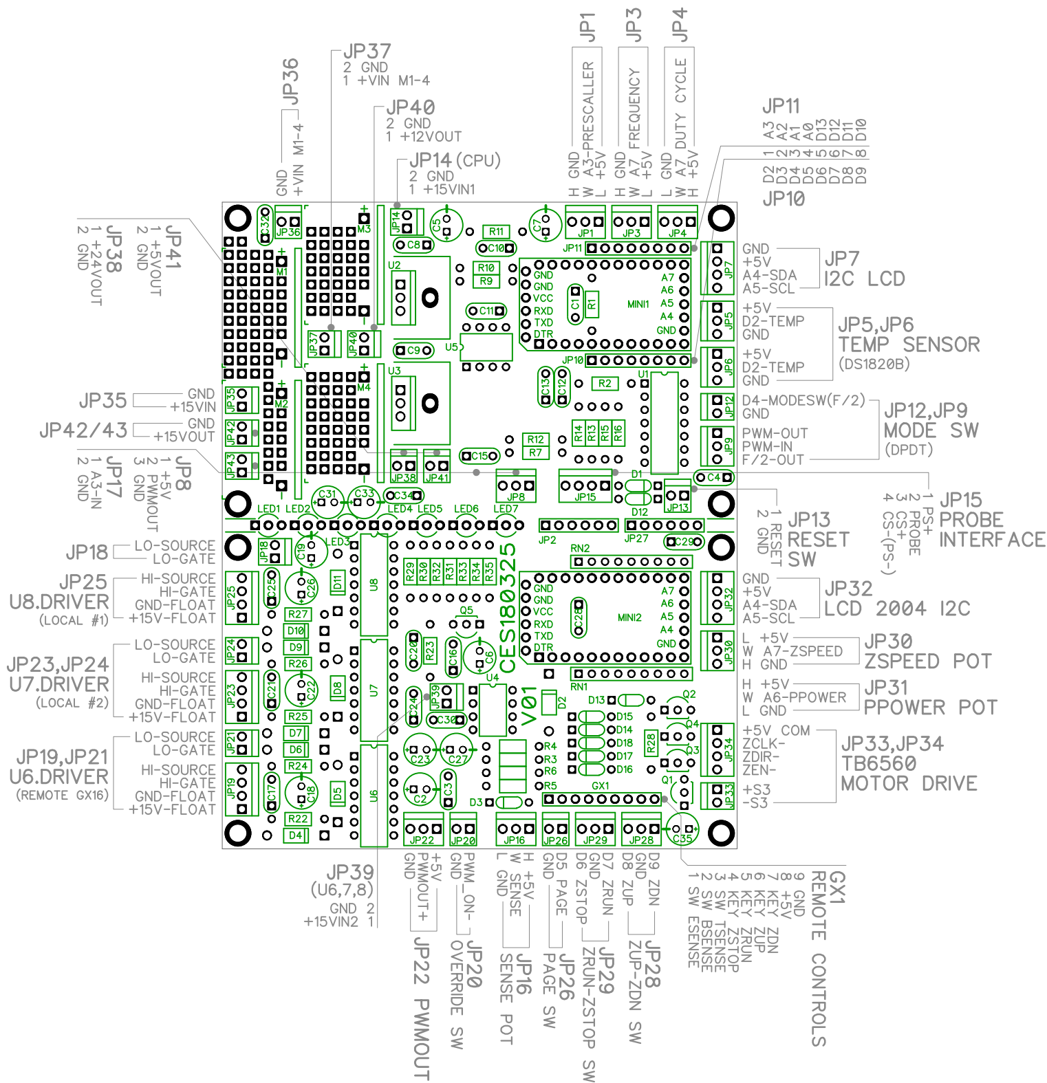
CES180325-1_v01 PCB ASSEMBLY
