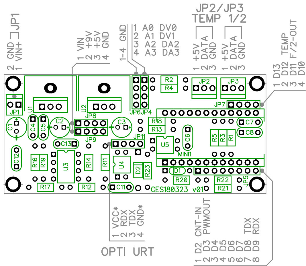
CES180323-3 PCB ASSY
