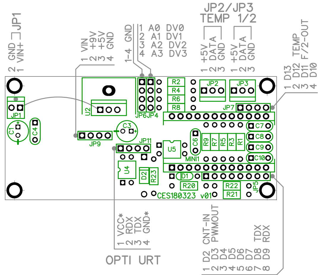
CES180323-2 PCB ASSY
